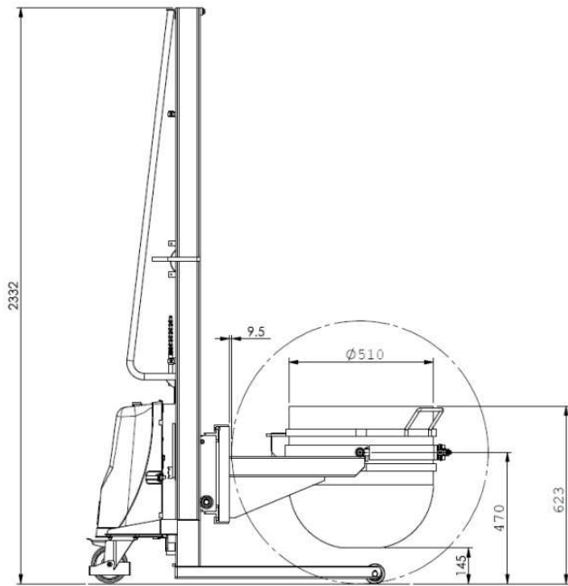
Sollevatore elettrico per vasche B100-160
